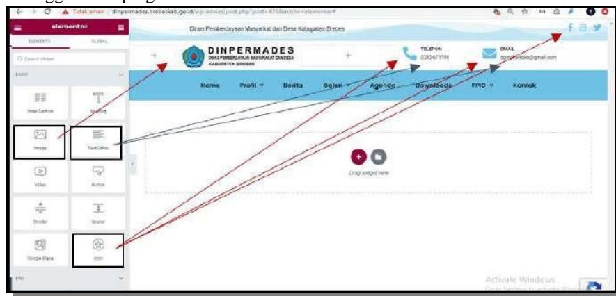
Gambar 9 Tampilan Header
