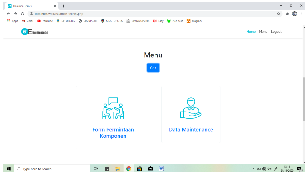
Gambar 2 Halaman Teknisi
