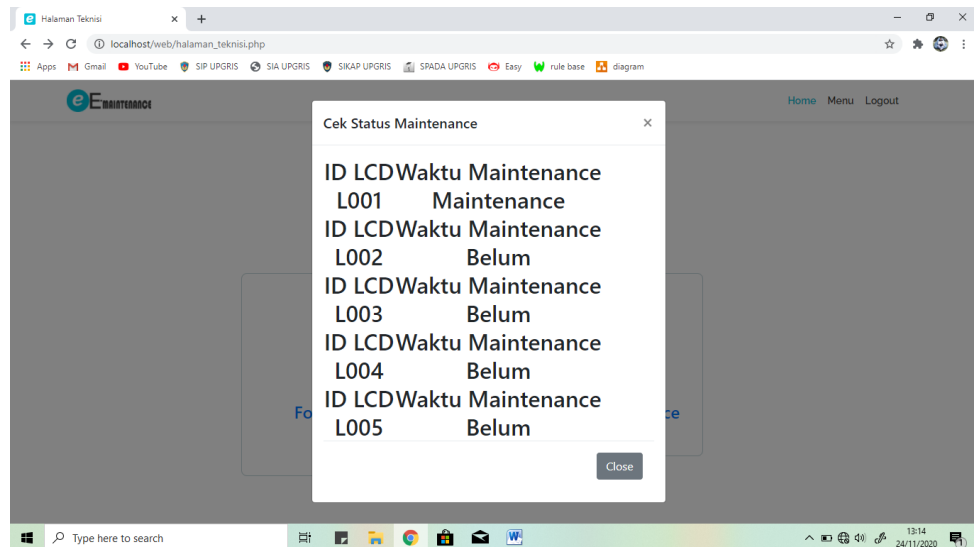
Gambar 3 Notifikasi Maintenance
