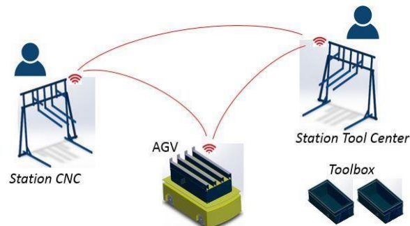
Gambar 2 gambaran umum perancangan sistem
