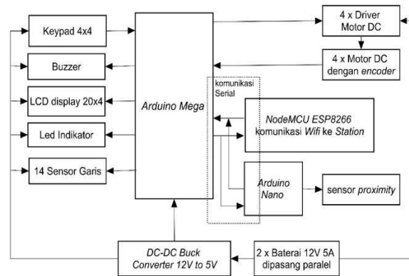
Gambar 6 blok diagram elektronika AGV
